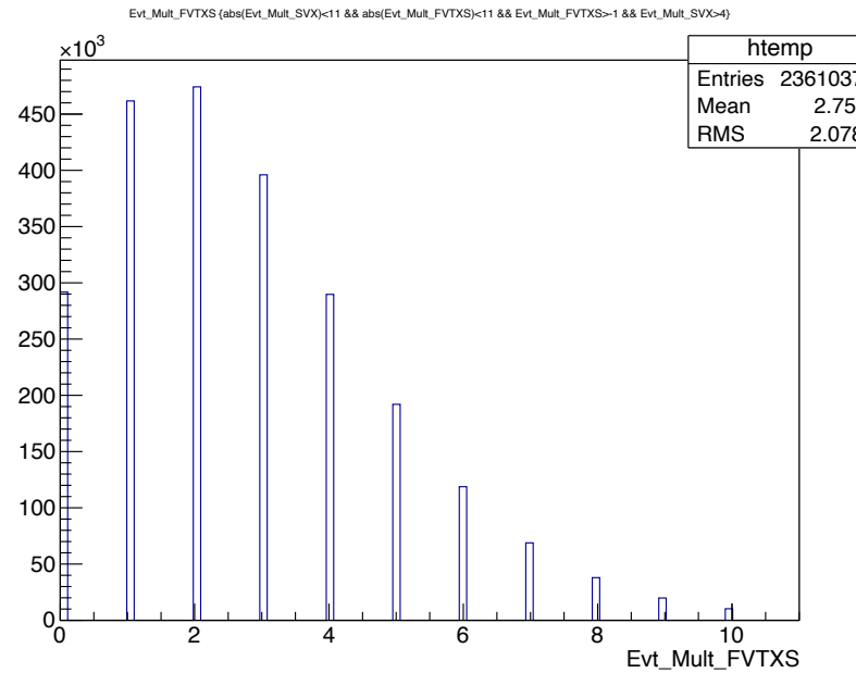
FVTXS_MB, SVX>4
