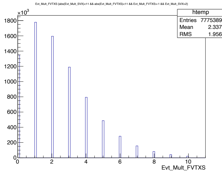
FVTXS_MB, SVX>2
