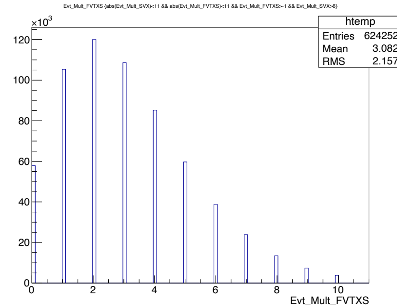
FVTXS_MB, SVX>6
