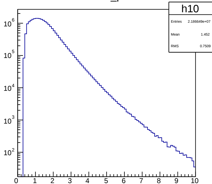
muon_pT
