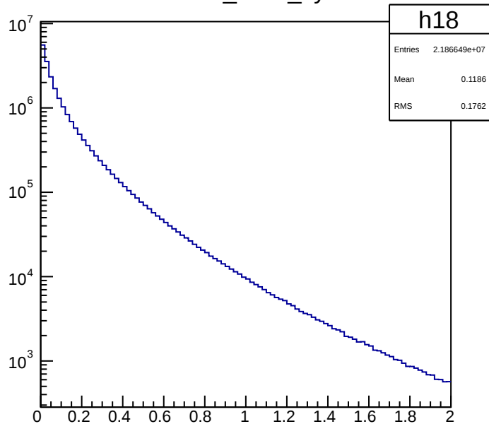
muon_DCA_xy
