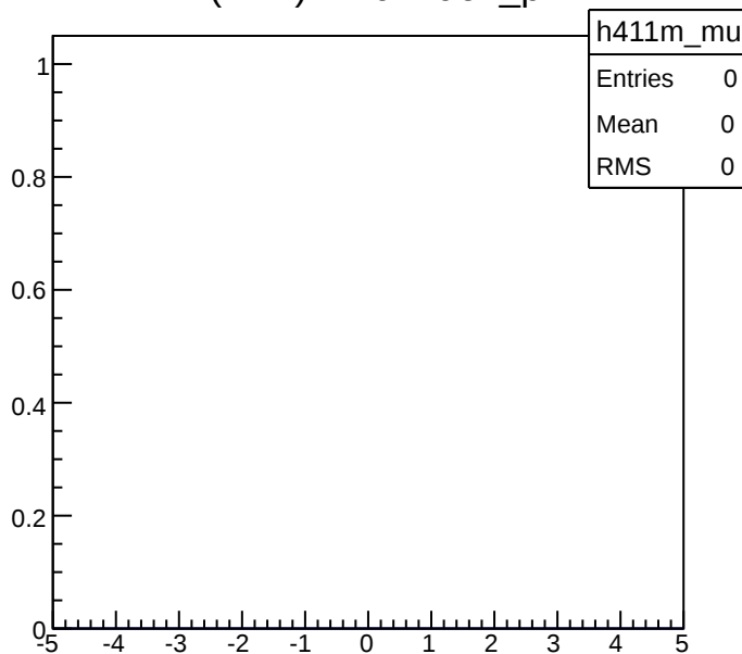
D-(-411)-&gt;mu muon_phi
