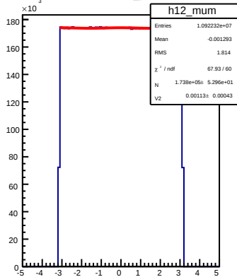
mu-: muon_phi
