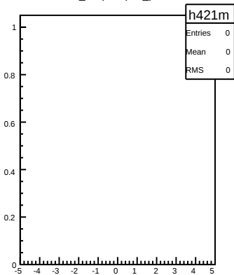
D0_bar(-421) D_phi
