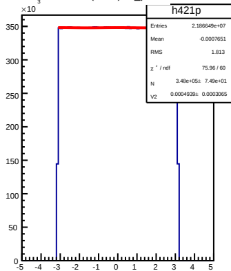
D0(+421) D_phi
