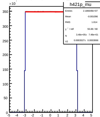
D0(+421)-&gt;muon_phi
