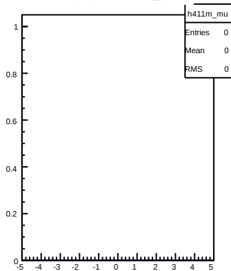
D-(-411)-&gt;muon_phi
