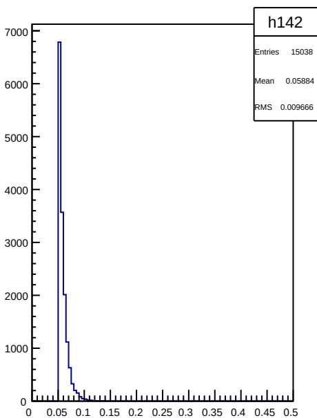
muon_xF
