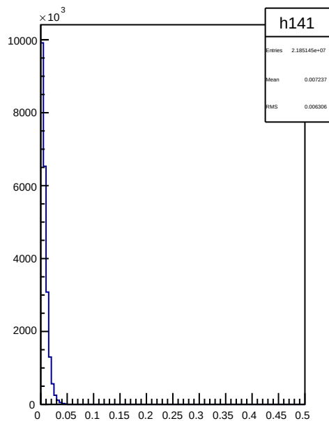
muon_xF
