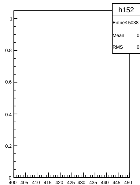
muon_PID
