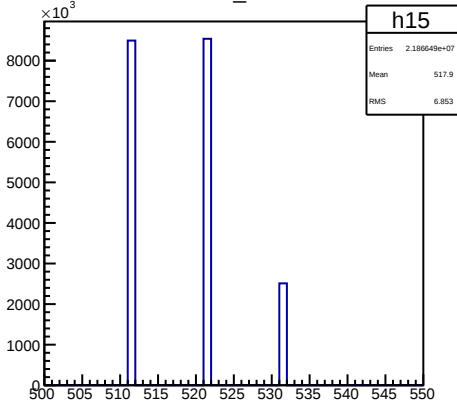
muon_PID
