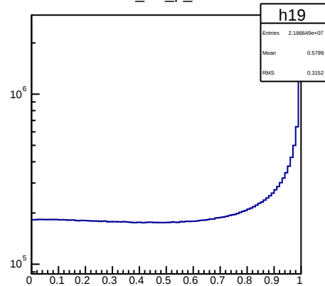
muon_vtx_p_sinXY
