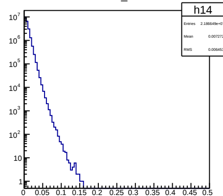
muon_xF
