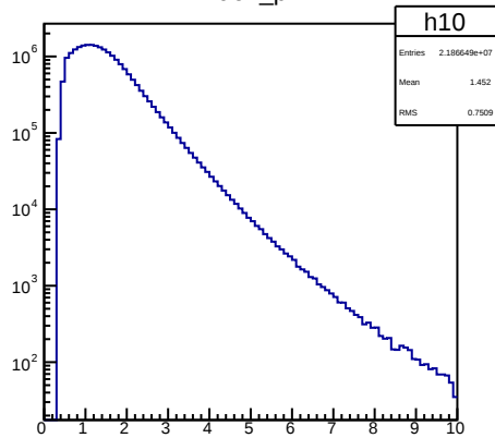
muon_pT
