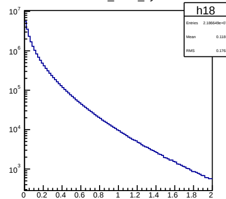
muon_DCA_xy
