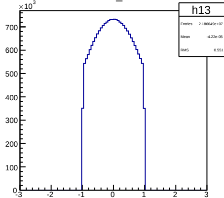
muon_eta
