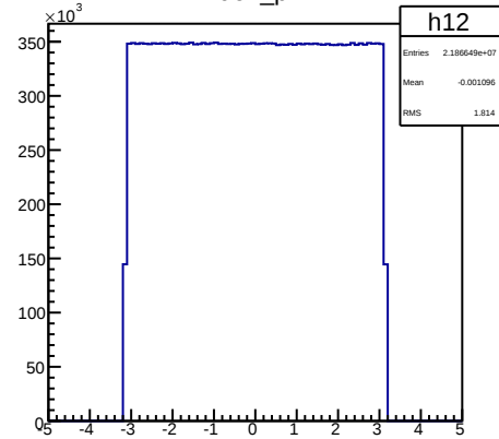
muon_phi
