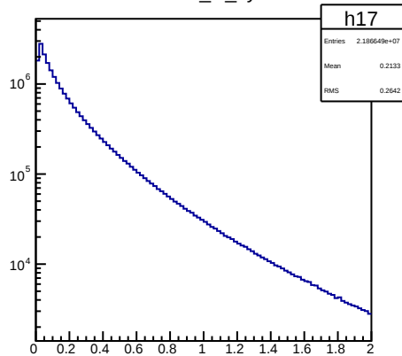
muon_R_xy
