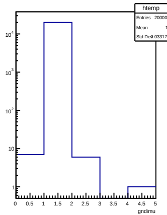
gndimu
