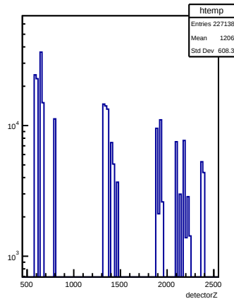
detectorZ
