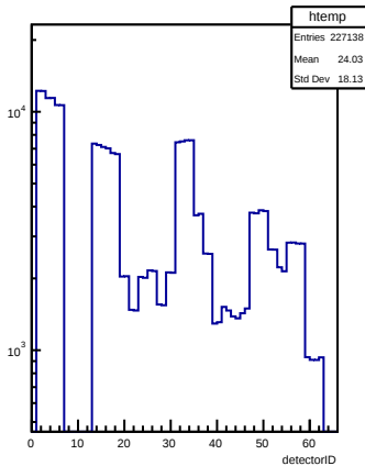
detectorID
