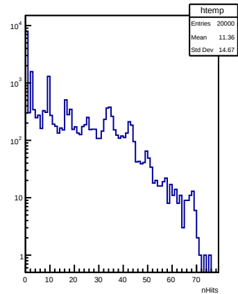
nHits
