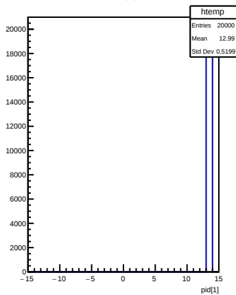
pid[1]
