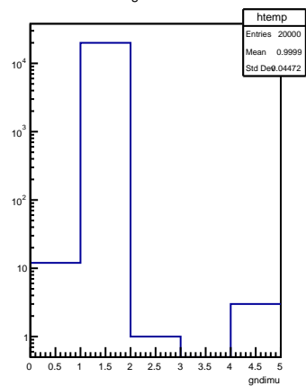
gndimu
