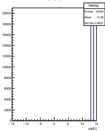
pid[1]
