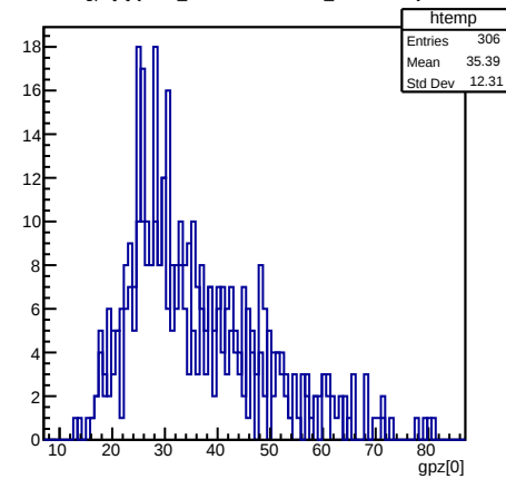
gpz[0] {dimu_mass&lt;10 &amp;&amp; dimu_mass &gt; 0.5}
