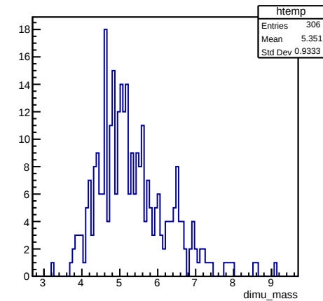
dimu_mass {dimu_mass&lt;10 &amp;&amp; dimu_mass &gt; 0.5}
