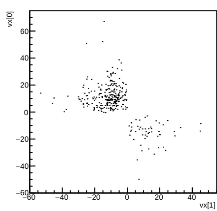
vx[0]:vx[1] {dimu_mass&lt;10 &amp;&amp; dimu_mass &gt; 0.5}
