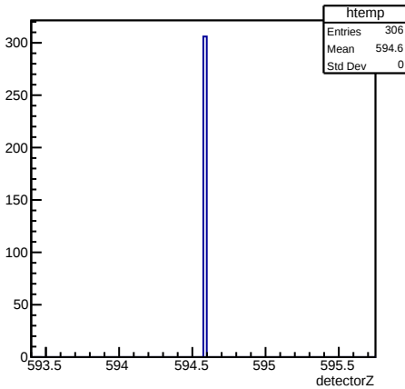
detectorZ {dimu_mass&lt;10 &amp;&amp; dimu_mass &gt; 0.5}
