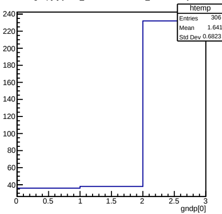
gndp[0] {dimu_mass&lt;10 &amp;&amp; dimu_mass &gt; 0.5}
