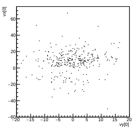
vx[0]:vy[0] {dimu_mass&lt;10 &amp;&amp; dimu_mass &gt; 0.5}
