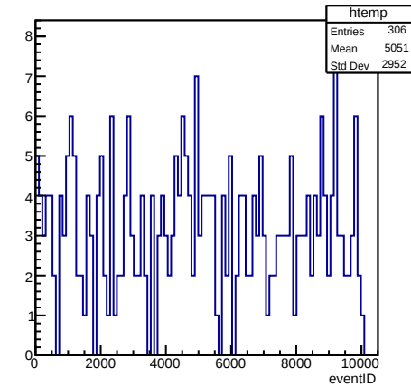
eventID {dimu_mass&lt;10 &amp;&amp; dimu_mass &gt; 0.5}
