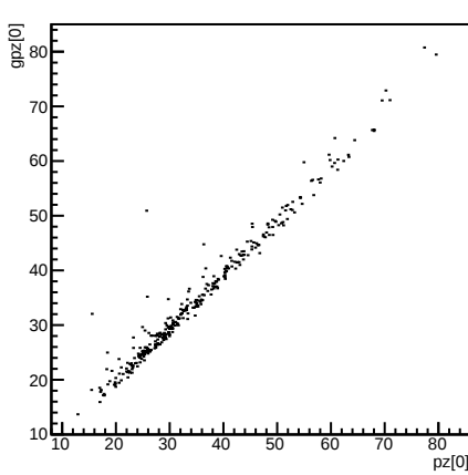
gpz[0]:pz[0] {dimu_mass&lt;10 &amp;&amp; dimu_mass &gt; 0.5}
