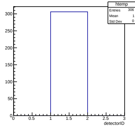
detectorID {dimu_mass&lt;10 &amp;&amp; dimu_mass &gt; 0.5}
