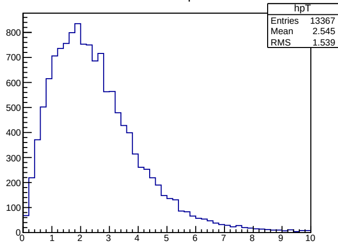
Drell-Yan pT
