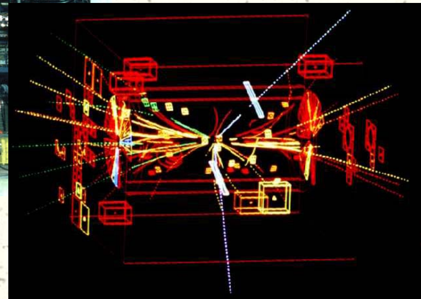
Premier Z^0 dans UA1
