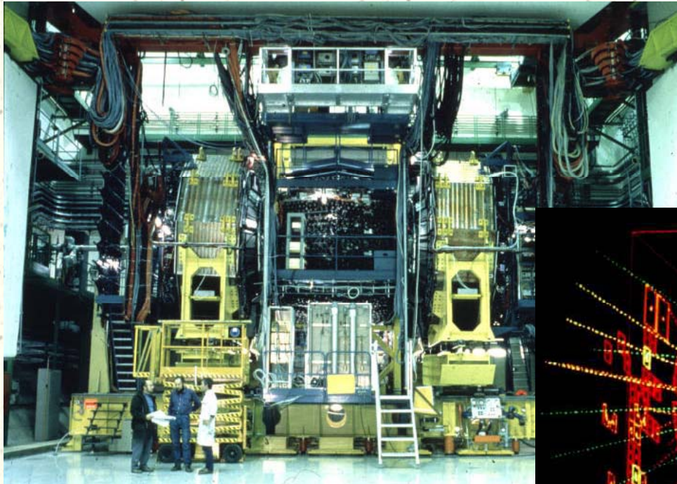
Expérience UA2
