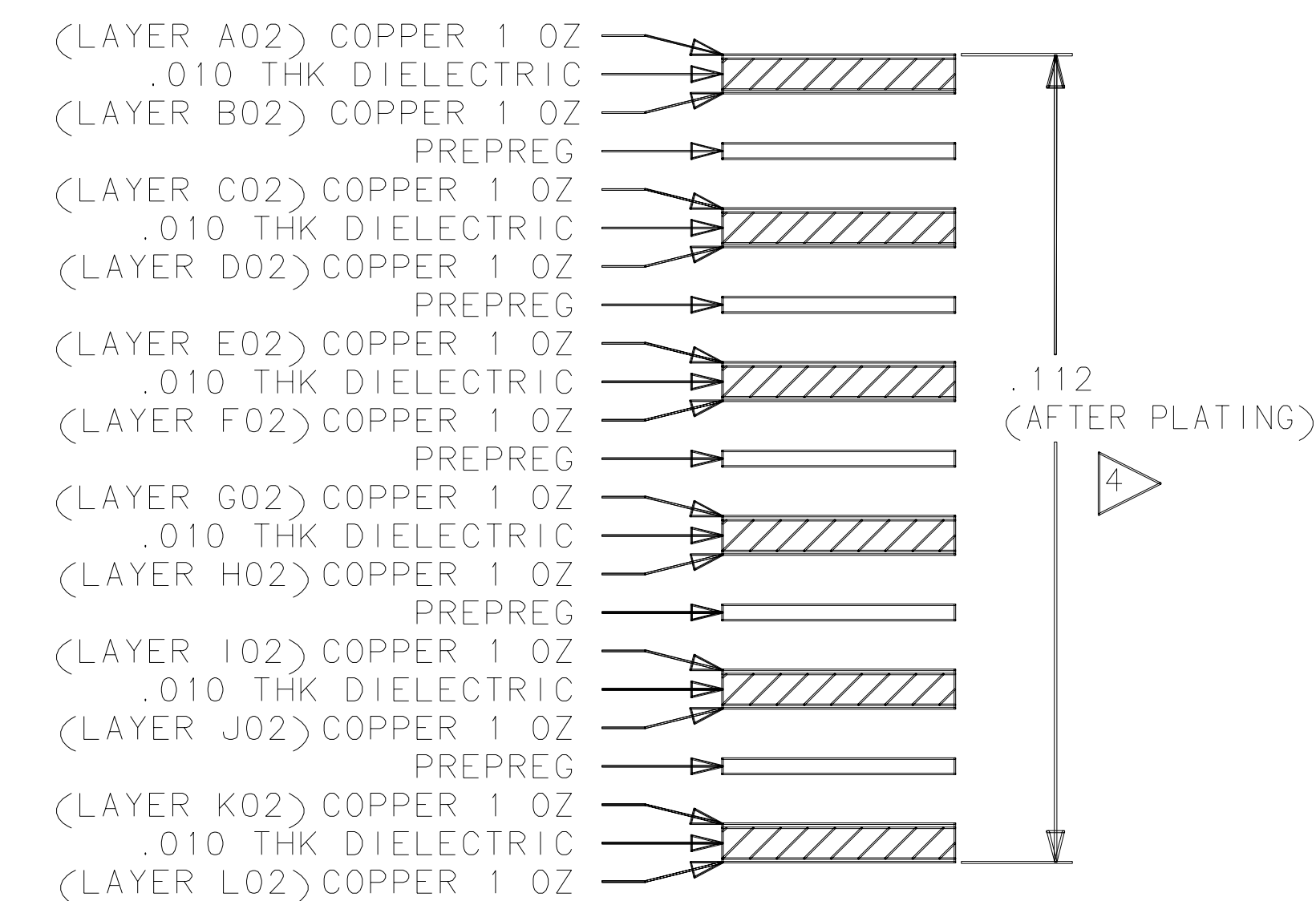
DETAIL 'A' 12 LAYER
